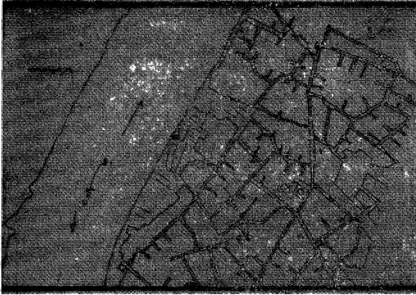
شكل - ٦
