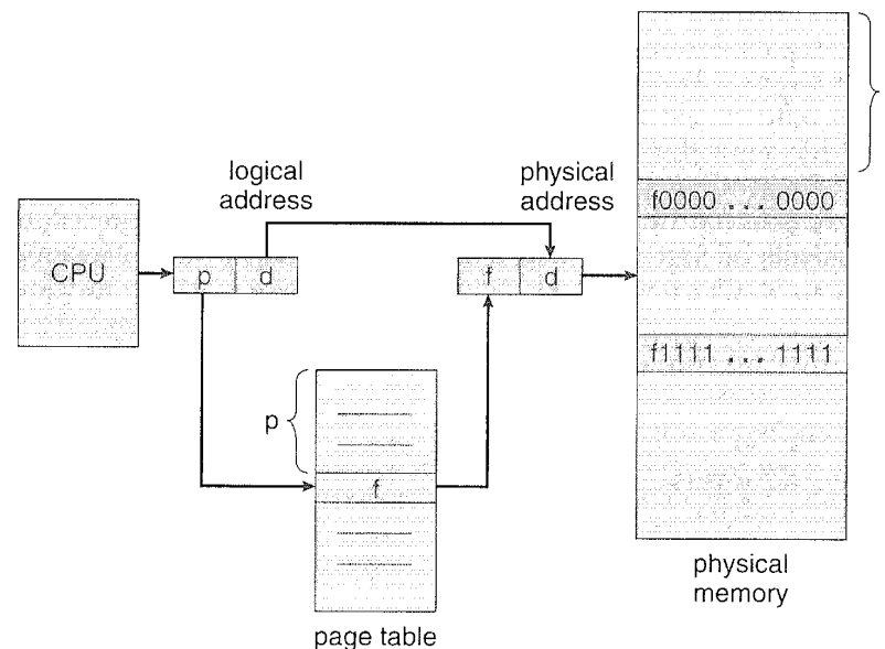
Figure 8.7 Paging hardware.
