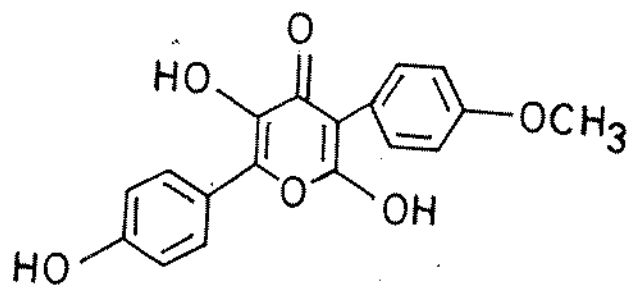
A - 1 - Pyrone deriv. (342)
