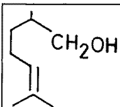
Citronellol (299)
