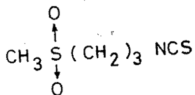
Cherirolin (72)
