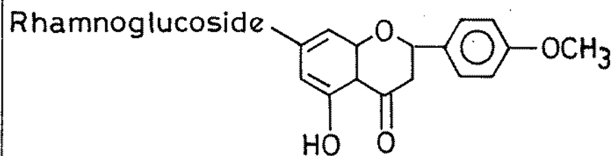
Citronin (82)
