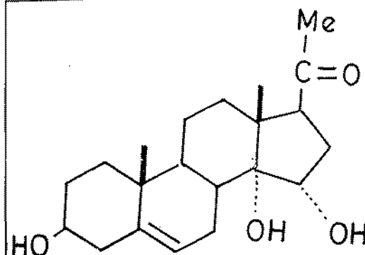
Purpnigenin (128)
