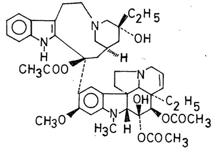
Vinrosidine, Leurosidine (352)
