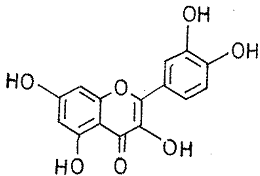
Quercetin (287 - 288)
