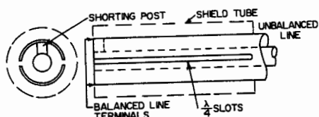
TYPE 10a SPLIT-TUBE BALUN
