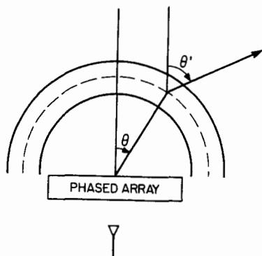
FIG. 16-19 Dome-antenna nomenclature.
