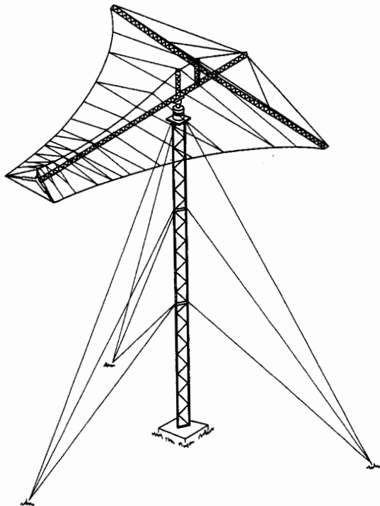
FIG. 26-12 Rotatable LPA.
