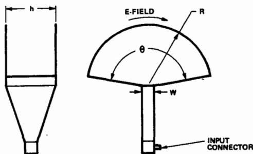
FIG. 40-1 E -plane radial-mode horn.
