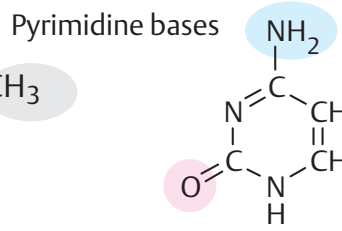
Cytosine (Cyt)
