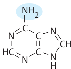
Adenine (Ade)
